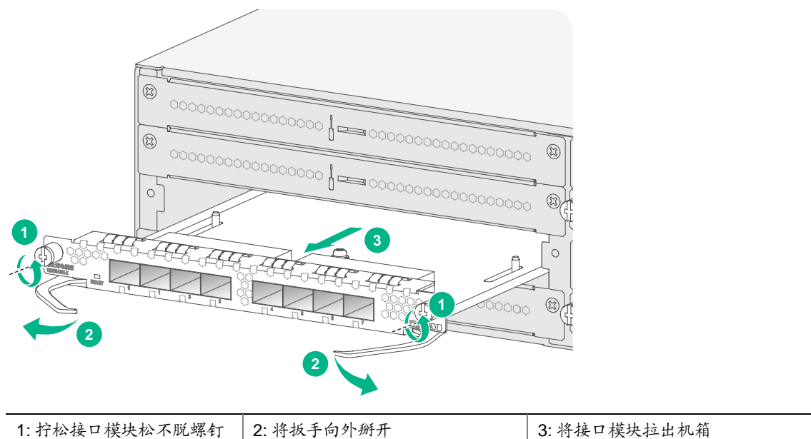
图4-4 拆卸接口模块
