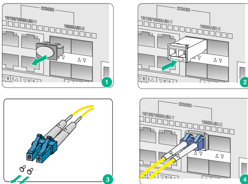
图2-14 安装及连接光模块
