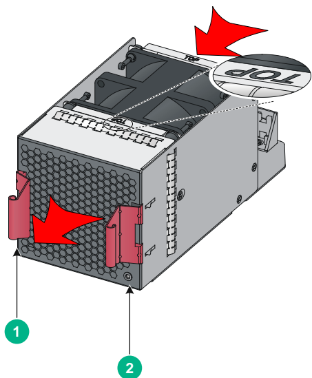
图A-12 FAN-20B-2-A
