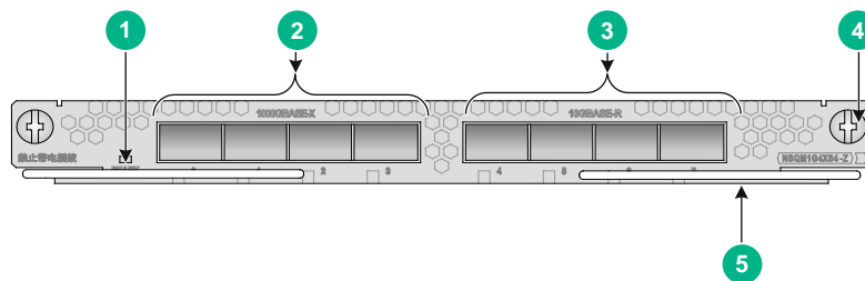
图A-5 NSQM1G4XS4-Z 接口模块正视图
