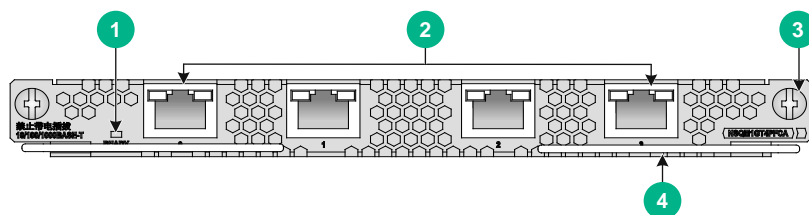
图A-8 NSQM1GT4PFCA 接口模块正视图
