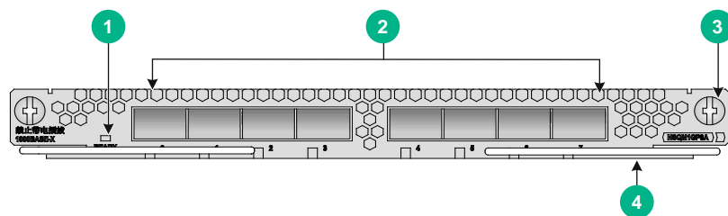
图A-7 NSQM1GP8A 接口模块正视图
