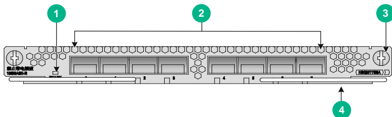
图A-3 NSQM1TG8A 接口模块正视图
