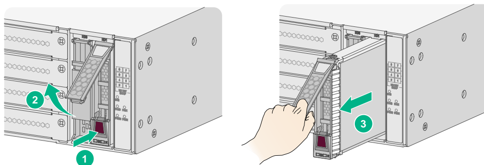
图2-10 拆卸硬盘
