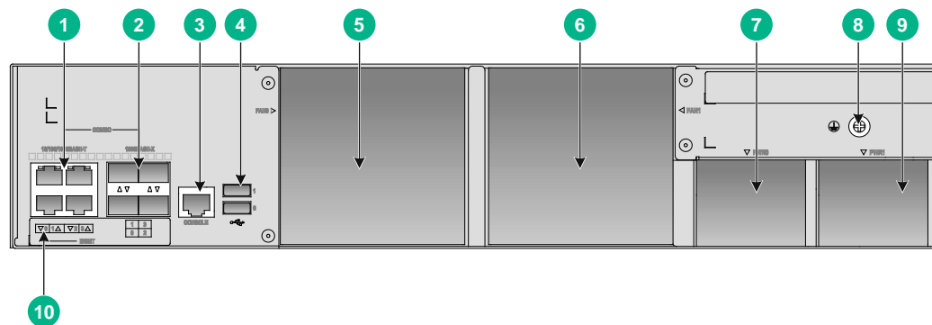
图A-2 设备后视图
