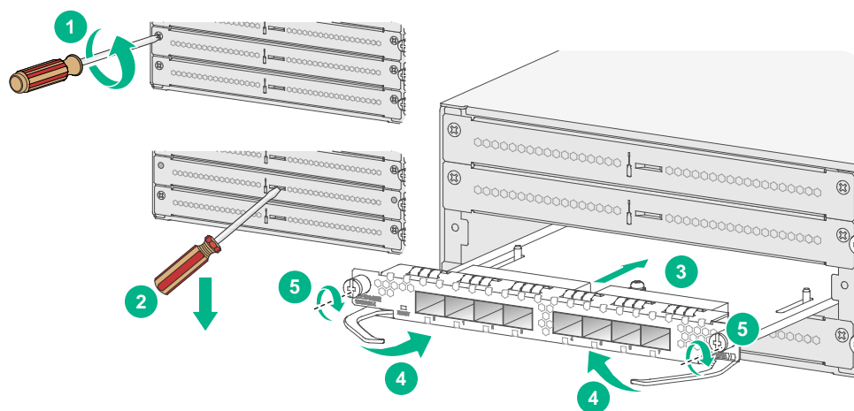
图2-8 安装接口模块
