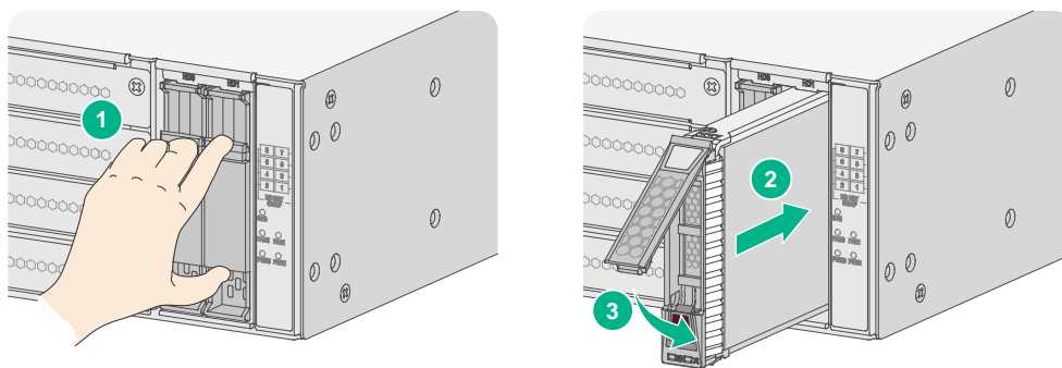
图2-9 安装硬盘
