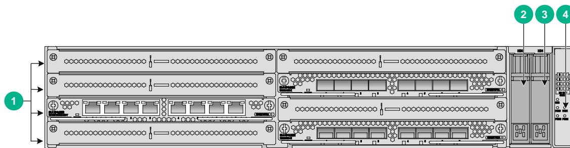
图A-1 设备前视图
