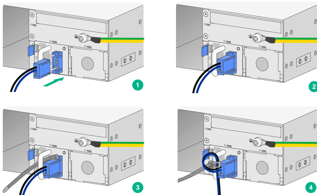
图2-16 连接直流电源线
