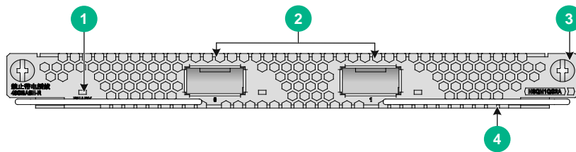
图A-4 NSQM1QG2A 接口模块正视图
