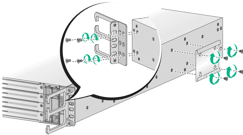
图2-2 安装前挂耳
