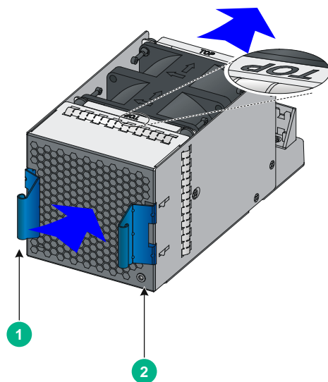
图A-11 FAN-20F-2-A
