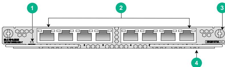
图A-6 NSQM1GT8A 接口模块正视图
