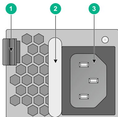
图A-9 交流电源模块正视图
